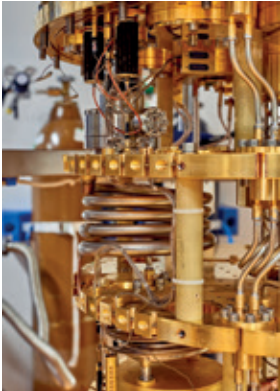
FOTO COVER Zeer geavanceerde koelinstallatie ‘cryostaat’ waarin qubits afgekoeld worden tot -273°C. Bij deze extreem lage temperaturen blijven de qubits lang genoeg in een quantumtoestand om er berekeningen mee uit te kunnen voeren.
